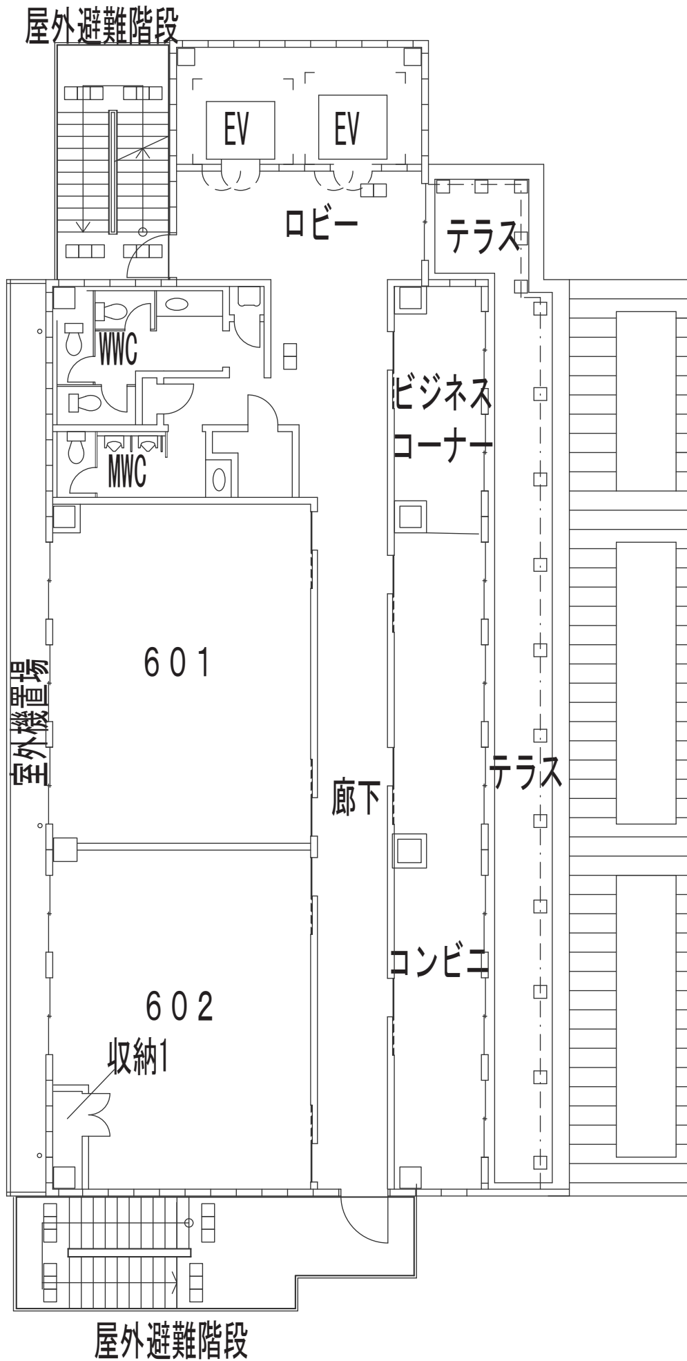
6階平面図
